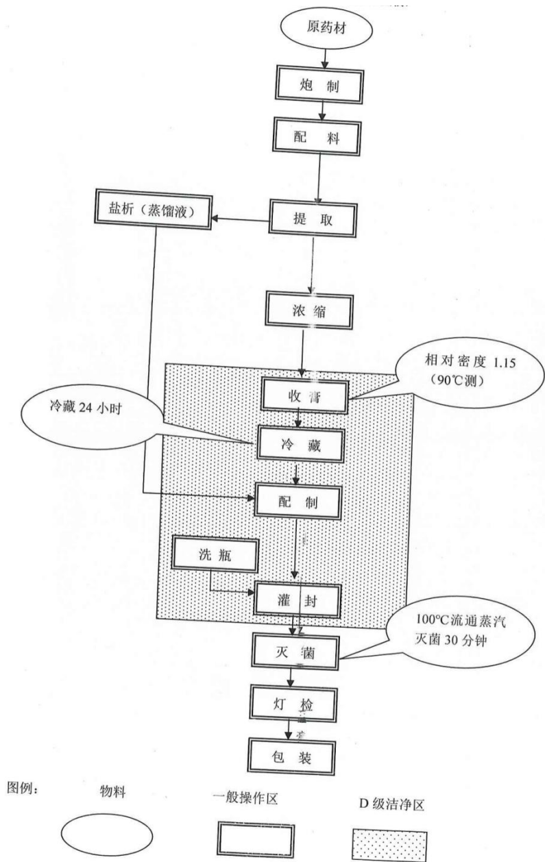
图 2.2 柴胡口服液工艺流程图
